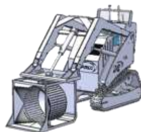
Sejalna žlica. Rotacija ločuje odpadke od vrhnje plasti zemlje.
